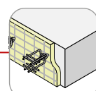
Mit Querkraftübertragung
