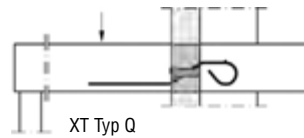
Schöck Isokorb® XT Typ Q positive Querkraft
