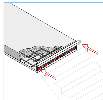
Egcostep® NG S8
