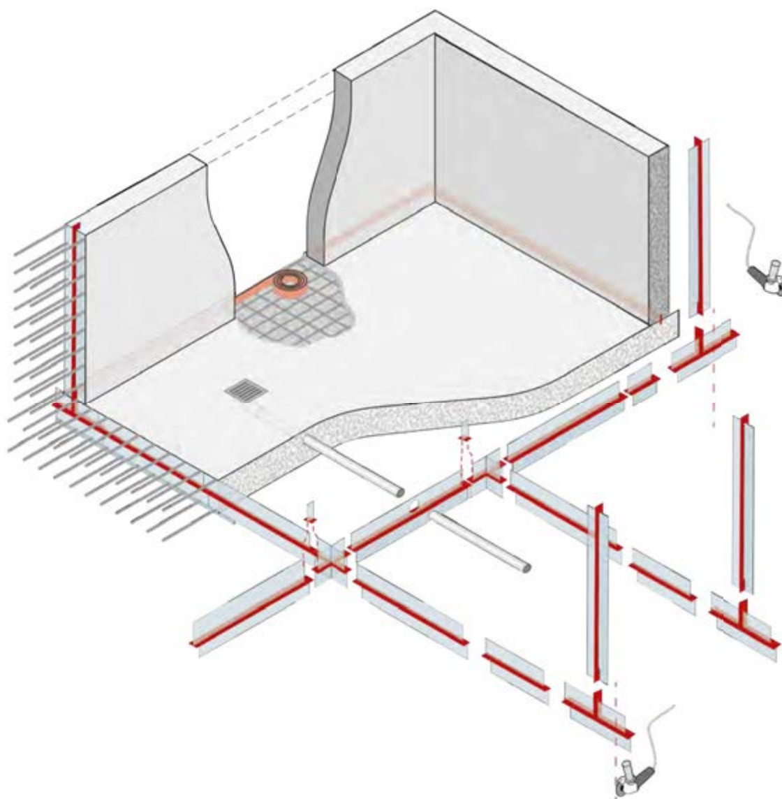
Eck-Formteil
